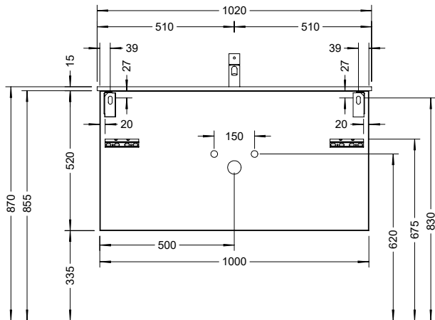
SFGP/SFGR/SFGT102
